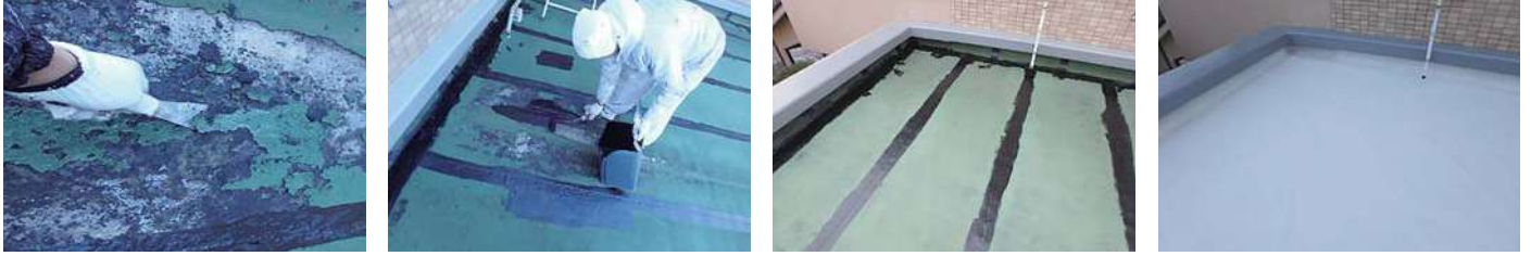
159 物件名 ▶ カサベリヤ菊地(豊島区北大塚) 施工期日: 令和5年12月 / 施工内容: 5階廊下漏水補修工事
