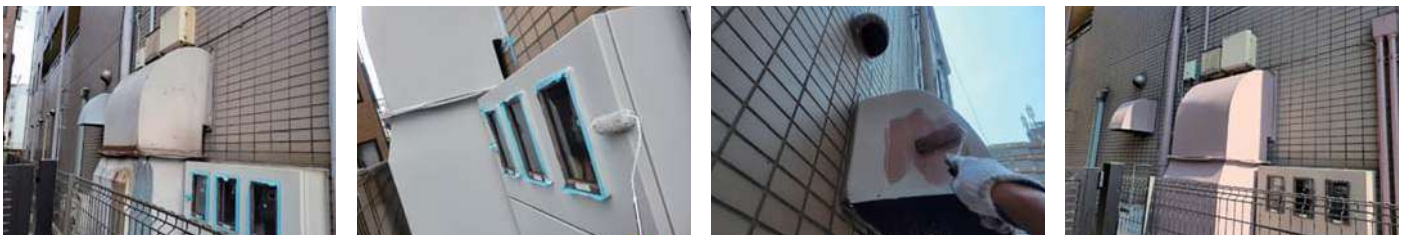
54 物件名▶ベルテックスビル(北区滝野川) 施工期日: 令和7年6月 / 施工内容: 塔屋漏水箇所調査補修工事
