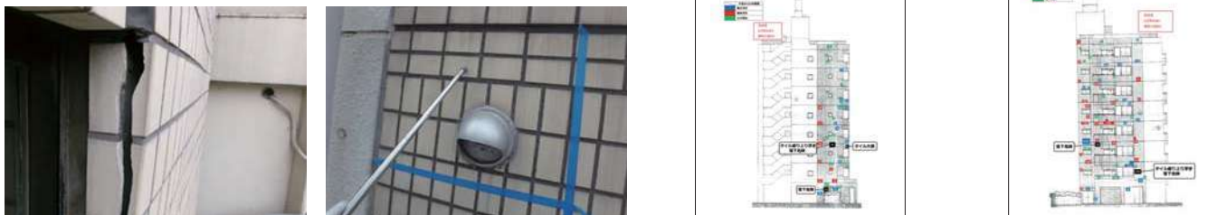
36 物件名 ▶ フリーデンカナメ(豊島区池袋) 施工期日: 令和7年5月 / 施工内容: タイル外壁打診調査
