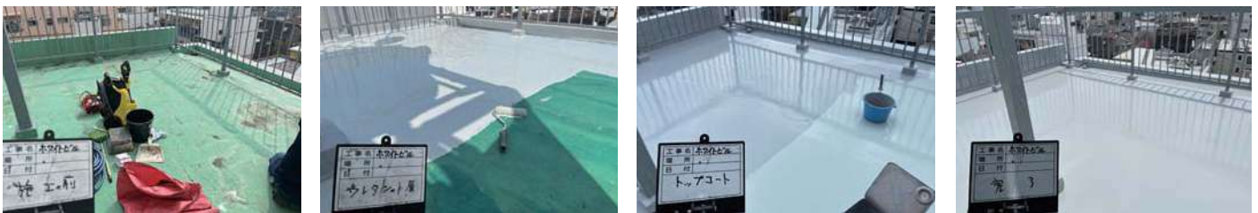
71 物件名 ▶ 細川ビル(港区赤坂) 施工期日: 令和7年7月 / 施工内容: 両妻面外壁塗装・屋上防水工事
