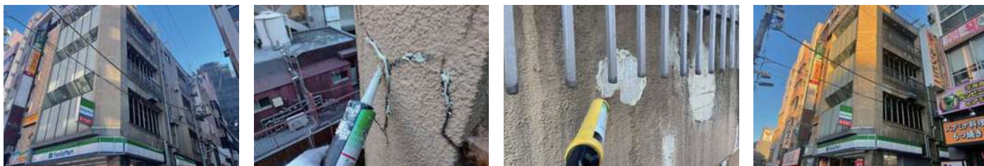
131 物件名 ▶ 細川ビル(港区赤坂) 施工期日: 令和7年12月 / 施工内容: 1階回り床左官補修工事
